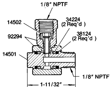
83822 SWIVEL
